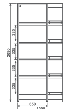
EC NF Expositor Canto Nacional Frio
