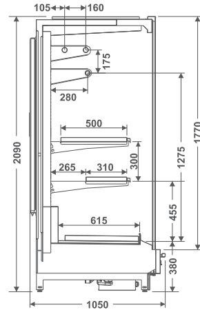
EVTVAG Expositor Vertical Vision Açougue Gancheira
