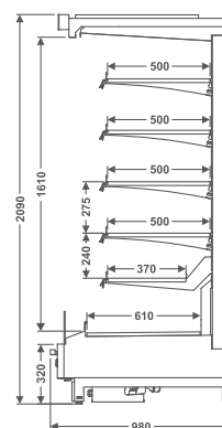
EVTVLA Expositor Vertical Vision Largo Aberto
