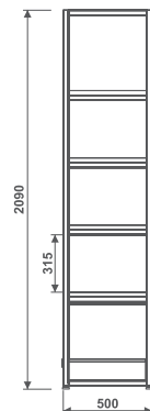
AP NF Adega Prateleira Nacional Frio
