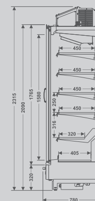
EVTVE PI Expositor Vertical Vision Estreito Plug-in
