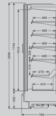
EVTVE CG Expositor Vertical Vision Estreito Congelados
