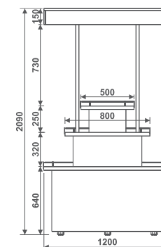
EDC NF Expositor Defumados Central Nacional Frio
