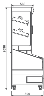
APTA NF Armário de Pães Tulha Alto Nacional Frio
