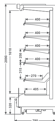
EVTVEA Expositor Vertical Vision Estreito Aberto
