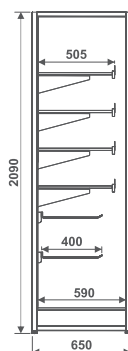
ET NF Expositor Temperos Nacional Frio
