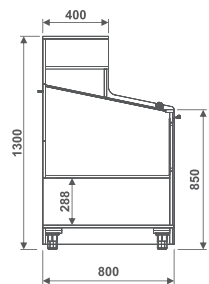
APTB NF Armário de Pães Tulha Baixo Nacional Frio
