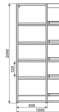
EC NF Expositor Canto Nacional Frio
