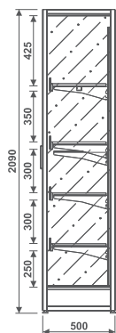
ACON NF Adega Confinados Nacional Frio
