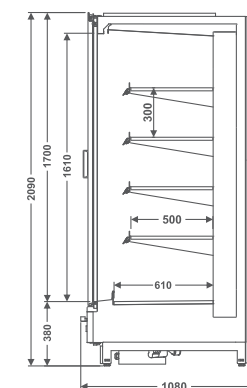
EVTV A Expositor Vertical Vision Atacado
