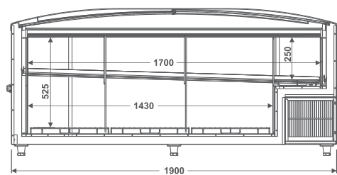
EISCT Expositor Ilha Skin Condenser Terminal
