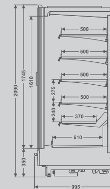
EVTVL CG Expositor Vertical Vision Largo Congelados
