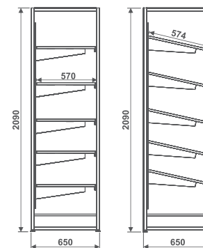
EPR NF Expositor Prateleira Regulável Nacional Frio
