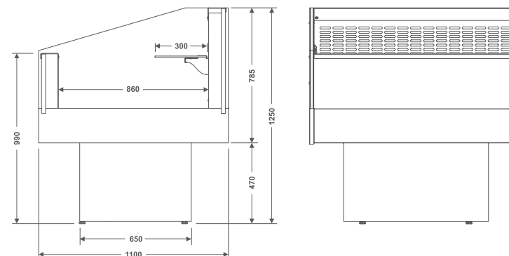
EHVP Expositor Horizontal Vision Prateleira
