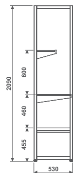
EG NF Expositor para Grãos Nacional Frio
