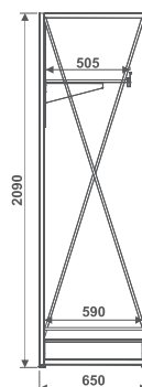
ECA NF Expositor Carvão Nacional Frio
